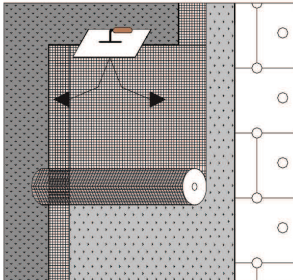
Obr. 34 Aplikace základní vrstvy
