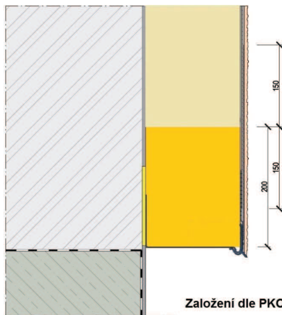
Varianty založení kontaktního zateplení (ETICS) dle ČSN 73 0810
