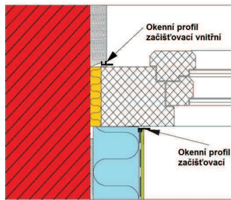
Obr. 20 Styk zateplení s okenním rámem řešený použitím okenního zajišťovacího profilu
