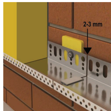
Obr. 5 Napojení základacích lišt s použitím spojek a vyrovnání nerovností zdiva pomocí distančních podložek
