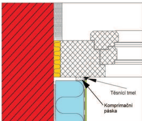
Obr. 19 Styk zateplení s okenním rámem řešený použitím pružného tmelu (starší způsob aplikace - již se nesmí provádět)
