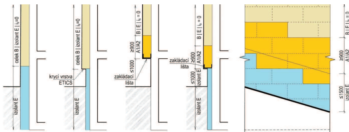
Varianty založení kontaktního zateplení (ETICS) dle ČSN 73 0810
