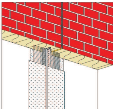
Obr. 17 Použití průběžného dilatačního profilu
