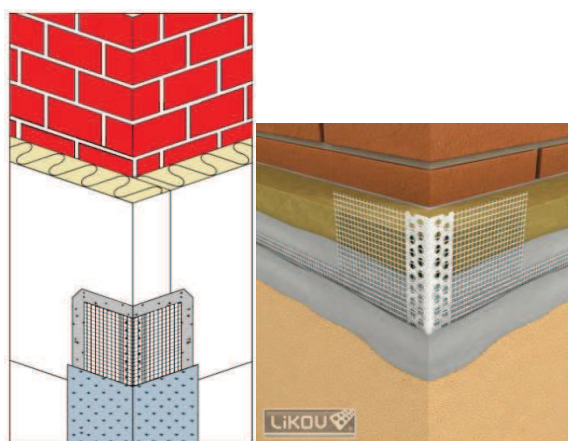
Obr. 28 Vyztužení nároží pomocí rohového profilu s integrovanou tkaninou (kombilišty) - pohled
