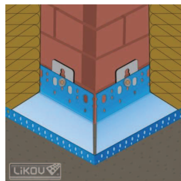
Obr. 7 Založení základací lišty na nároží
