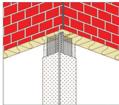
Obr. 18 Použití rohového dilatačního profilu
