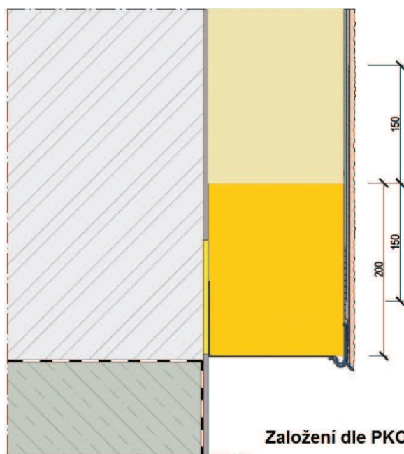
Varianty založení kontaktního zateplení (ETICS)
