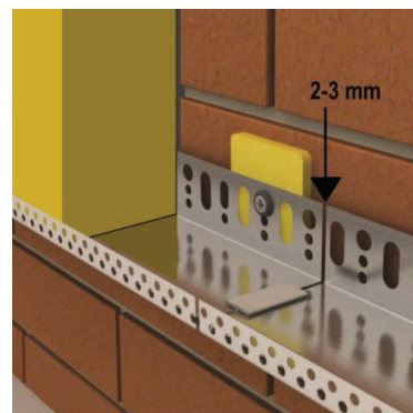
Obr. 5 Napojení základacích lišt s použitím spojek a vyrovnání nerovností zdíva pomocí distančních podložek
