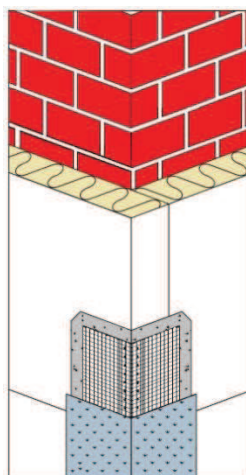
Obr. 28 Vyztužení nároží pomocí rohového profilu s integrovanou tkaninou (kombilišty) - pohled
