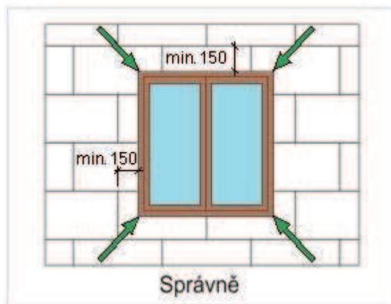
Obr. 12 Lepení desek izolantu u otvorových výplní
