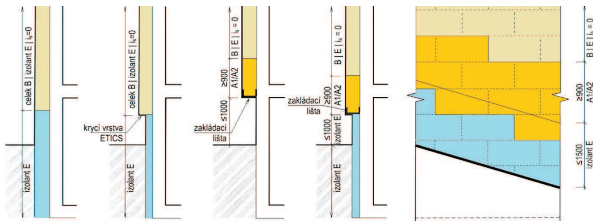
Varianty založení kontaktního zateplení (ETICS)
