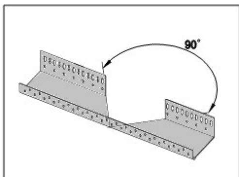
Obr. 6 Příprava základací lišty pro založení na nároží
