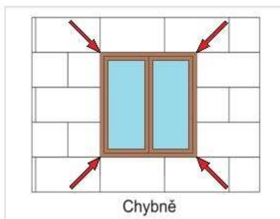
Obr. 11 Lenění desek izolantu u otvorových vlní
