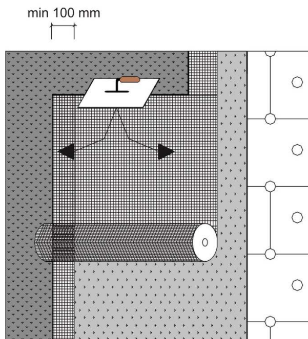
Obr. 32 Aplikace základní vrstvy
