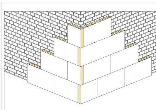
Obr. 10 Lepení desek izolantu na vazbu s provázáním na
