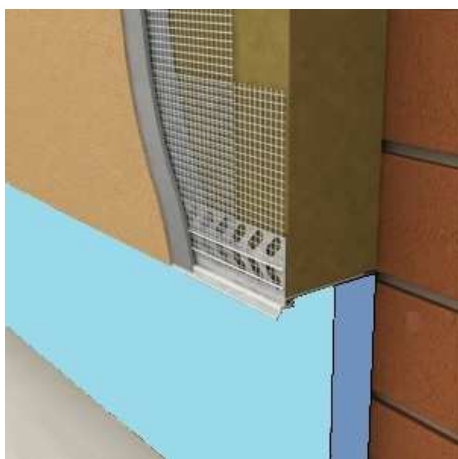
Obr. 21 Založení soklového profilu při zateplení soklu (ukončení pod terémem)
