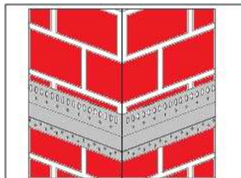
Obr. 7 Založení základací lišty na nároží
