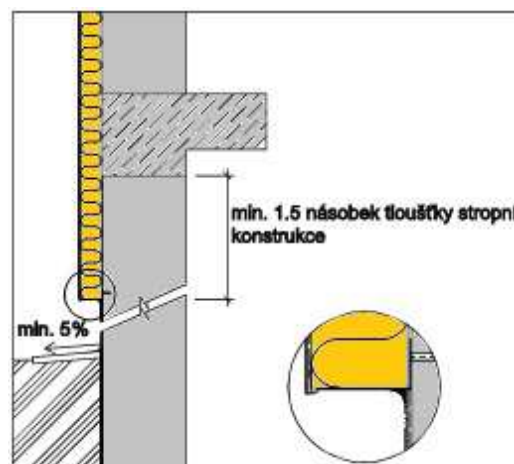
Obr. 4 Založení zakládacích lišt (varianta bez zateplení soklu)
