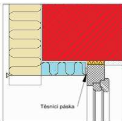
Obr. 12 Zakládání izolantu v ostění (vodorovný řez)
